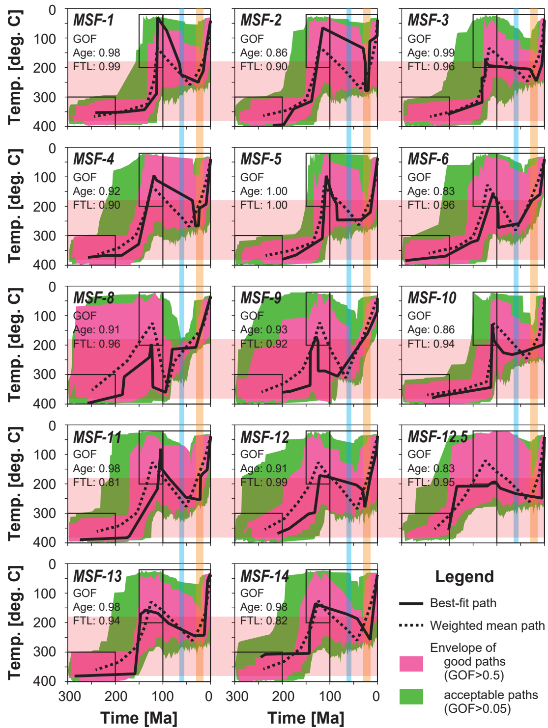
図2 熱史逆解析の結果. GOFはgoodness of fitの略で, FT年代とFT長分布のモデル値と実測値の適合度を表す (Ketcham, 2005). 水色とオレンジの縦帯は, 神岡鉱床形成 (65~55Ma) と日本海拡大 (30~15Ma) のおよその時期を示す. 薄赤の横帯は, ZFT系の準安定領域 (partial annealing zone; 180~380°C) を表す.
